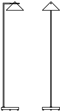
LUMINÁRIA 28 X 24 X 148 cm (LxPxA)
