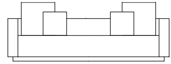
SOFÁ 240 X 130 X 63 cm (LxPxA) Almofadas: 02 unidades decorativas 60x60 cm com faixa 02 unidades decorativas 100x100 cm
