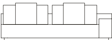
SOFÁ 260 X 100 X 63 cm (LxPxA) Almofadas: 02 unidades decorativas 60x60 cm 02 unidades de encosto 02 unidades rolinho de encosto (L = 105 cm)
