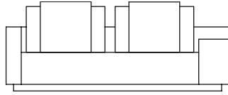
SOFÁ 220 X 100 X 63 cm (LxPxA) Almofadas: 02 unidades decorativas 60x60 cm 02 unidades de encosto 02 unidades rolinho de encosto (L = 90 cm)
