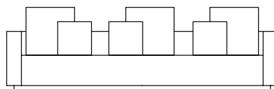
SOFÁ 280 X 160 X 63 cm (LxPxA) Almofadas: 03 unidades decorativas 60x60 cm com faixa 03 unidades decorativas 100x100 cm
