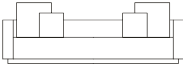
SOFÁ 260 X 130 X 63 cm (LxPxA) Almofadas: 02 unidades decorativas 60x60 cm com faixa 02 unidades decorativas 100x100 cm
