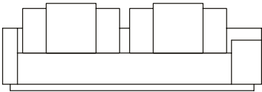
SOFÁ 260 X 100 X 63 cm (LxPxA) Almofadas: 02 unidades decorativas 60x60 cm 02 unidades de encosto 02 unidades rolinho de encosto (L = 110 cm)
