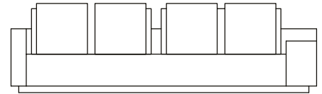
SOFÁ 300 X 100 X 63 cm (LxPxA) Almofadas: 03 unidades decorativas 60x60 cm 03 unidades de encosto 03 unidades rolinho de encosto (L = 83 cm)
