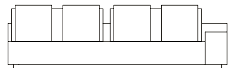
SOFÁ 300 X 100 X 63 cm (LxPxA) Almofadas: 04 unidades decorativas 60x60 cm 02 unidades de encosto 02 unidades rolinho de encosto (L = 125 cm)
