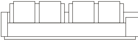
SOFÁ 320 X 100 X 63 cm (LxPxA) Almofadas: 03 unidades decorativas 60x60 cm 03 unidades de encosto 03 unidades rolinho de encosto (L = 90 cm)
