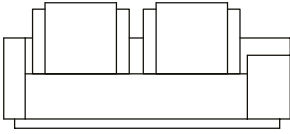
SOFÁ 200 X 100 X 63 cm (LxPxA) Almofadas: 02 unidades decorativas 60x60 cm 02 unidades de encosto 02 unidades rolinho de encosto (L = 80 cm)
