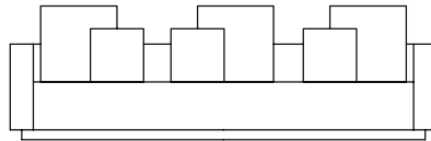
SOFÁ 280 X 130 X 63 cm (LxPxA) Almofadas: 03 unidades decorativas 60x60 cm com faixa 03 unidades decorativas 100x100 cm
