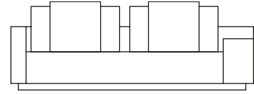
SOFÁ 240 X 100 X 63 cm (LxPxA) Almofadas: 02 unidades decorativas 60x60 cm 02 unidades de encosto 02 unidades rolinho de encosto (L = 100 cm)
