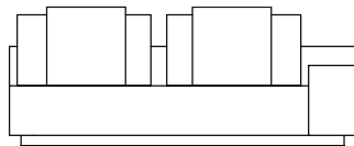
SOFÁ 220 X 100 X 63 cm (LxPxA) Almofadas: 02 unidades decorativas 60x60 cm 02 unidades de encosto 02 unidades rolinho de encosto (L = 85 cm)
