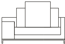
POLTRONA 150 X 100 X 61 cm (LxPxA) Almofadas: 01 unidade de encosto (L = 100 cm) 01 unidade de rolinho de encosto 01 unidade decorativa 60x60 cm
