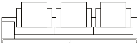
SOFÁ 320 X 100 X 61 cm (LxPxA) Almofadas: 03 unidades de encosto (L = 83 cm) 03 unidades de rolinho de encosto 03 unidades decorativas 60x60 cm
