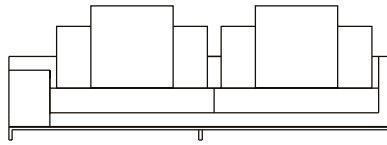
SOFÁ 280 X 100 X 61 cm (LxPxA) Almofadas: 02 unidades de encosto (L = 110 cm) 02 unidades de rolinho de encosto 02 unidades decorativas 60x60 cm
