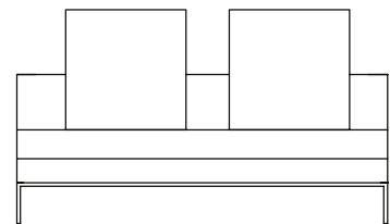
CHAISE 154 X 154 X 62 cm (LxPxA) Almofadas: 02 unidades decorativas 70x70 cm 01 unidade de assento (L = 154 cm) 01 unidade de encosto inteiriça (A = 34 cm)
