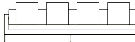
SOFÁ 300 X 110 X 62 cm (LxPxA) Almofadas: 04 unidades decorativas 70x70 cm 01 unidade de assento (L = 280 cm) 01 unidade de encosto e braço inteiriça (A = 34 cm)
