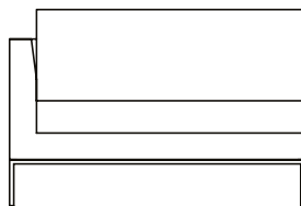
POLTRONA 1BR 110 X 110 X 62 cm (LxPxA) Almofadas: 01 unidade de assento (L = 100 cm) 01 unidade de encosto inteira (A = 34 cm)
