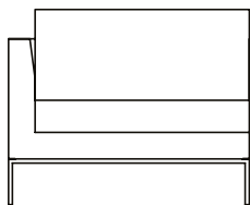
POLTRONA 1BR 90 X 90 X 62 cm (LxPxA) Almofadas: 01 unidade de assento (L = 80 cm) 01 unidade de encosto inteira (A = 34 cm)
