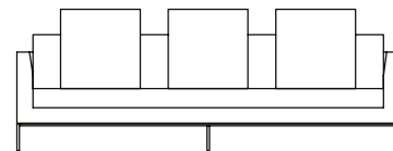
SOFÁ 240 X 110 X 62 cm (LxPxA) Almofadas: 03 unidades decorativas 70x70 cm 01 unidade de assento (L = 220 cm) 01 unidade de encosto e braço inteiriça (A = 34 cm)
