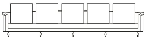
SOFÁ 360 X 110 X 70 cm (LxPxA) Almofadas: 01 unidade de assento (L = 341 cm) 05 unidades decorativas 60x60 cm
