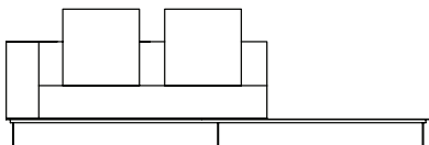
SOFÁ 260 X 100 X 64 cm (LxPxA) Almofadas: 02 unidades decorativas 60x60 cm 01 unidade de assento (L = 140 cm)
