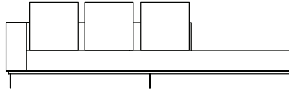
SOFÁ 280 X 100 X 64 cm (LxPxA) Almofadas: 03 unidades decorativas 60x60 cm 01 unidade de assento (L = 260 cm)
