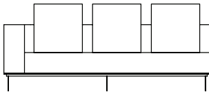
SOFÁ 200 X 100 X 64 cm (LxPxA) Almofadas: 03 unidades decorativas 60x60 cm 01 unidade de assento (L = 180 cm)
