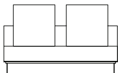
POLTRONA 150 X 100 X 64 cm (LxPxA) Almofadas: 02 unidades decorativas 60x60 cm 01 unidade de assento (L = 150 cm)
