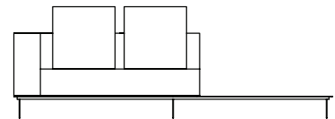
SOFÁ 240 X 100 X 64 cm (LxPxA) Almofadas: 02 unidades decorativas 60x60 cm 01 unidade de assento (L = 120 cm)
