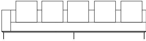
SOFÁ 320 X 100 X 64 cm (LxPxA) Almofadas: 05 unidades decorativas 60x60 cm 01 unidade de assento (L = 300 cm)
