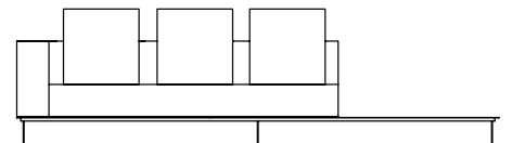
SOFÁ 300 X 100 X 64 cm (LxPxA) Almofadas: 03 unidades decorativas 60x60 cm 01 unidade de assento (L = 180 cm)
