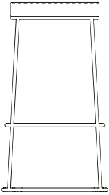
BANQUETA 42 X 37 X 74 cm (LxPxA)
