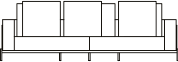
SOFÁ 260 X 95 X 63 cm (LxPxA) Almofadas: 03 unidades decorativas 60x60 cm
