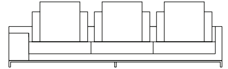
SOFA 320 x 100 x 61cm (LxPxA) Almofadas: 03 unidades de encosto (L=83cm) 03 unidades rolinho de encosto 03 unidades decorativa 60x60cm
