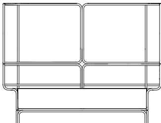
HIGHBACK 180 X 87 X 137cm (LxPxA) Almofadas: 05 unidades decorativas pastel 60x60cm 01 unidade de assento (146x70cm)
