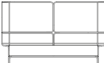
HIGHBACK 230 X 87 X 137cm (LxPxA) Almofadas: 06 unidades decorativas pastel 60x60cm 01 unidade de assento (196x70cm)
