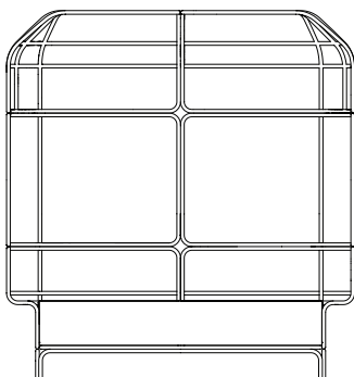
HIGHBACK TETO 180 X 87 X 190cm (LxPxA) Almofadas: 05 unidades decorativas pastel 60x60cm 01 unidade de assento (146x70cm)
