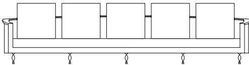
SOFA 360 x 127 x 70cm (LxPxA) Almofadas: 01 unidade de assento (L=341cm) 05 unidades decorativa 60x60cm
