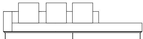
SOFÁ 320 X 100 X 64cm (LxPxA) Almofadas: 03 unidades decorativa 60x60cm 01 unidade de assento (L=300cm)
