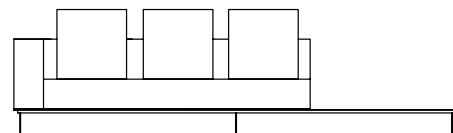
SOFÁ 300 X 100 X 64cm (LxPxA) Almofadas: 03 unidades decorativa 60x60cm 01 unidade de assento (L=180cm)
