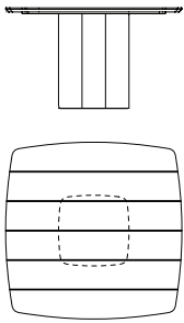
MESA JANTAR 130 X 130 X 74cm (LxPxA)
