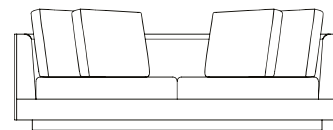
SOFA 220 x 95 x 65cm (LxPxA) Almofadas: 02 unidades de assento; 04 unidades decorativas 60x60cm com faixa
