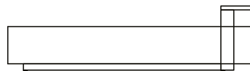
PUFE COM APOIO 190 X 070 X 52cm (LxPxA)
