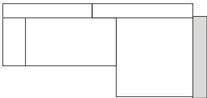
VISTA SUPERIOR (DIMENSÕES TOTAIS) 360 X 165 X 65cm (LxPxA)
